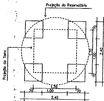
PLANTA BAIXA
