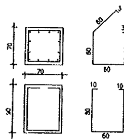
DETALHE FUNDAÇÕES
